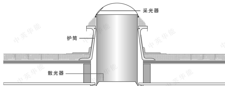
平顶安装节点图
