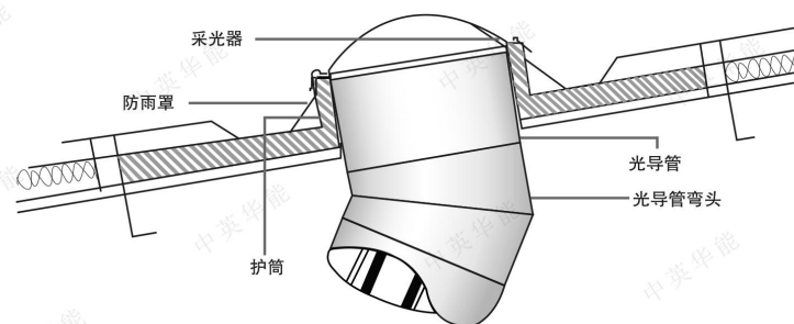
尖顶斜式安装节点图
